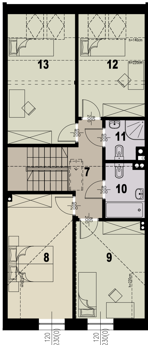
PODDASZE
